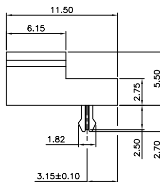
SECTION A-A 1:1
