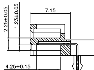
SECTION B-B 1:1
