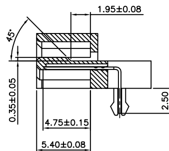
SECTION A-A 1:1
