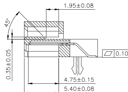
SECTION A-A 1:1
