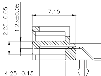
SECTION B-B 1:1
